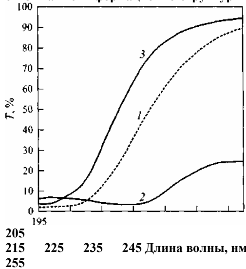
Рис. 4. Изменение УФ-спектра пропускания растворов \text{SnCl}_2 при химическом изменении кислотности: 2 — при добавлении щелочи (KOH), 3 — при добавлении кислоты (HCl); 1 — исходный раствор.
