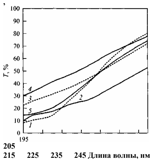
Рис. 3. Изменение УФ-спектра пропускания раствора \text{SnCl}_2 в результате пребывания в пирамиде в течение 5 часов на разных уровнях: 2 — на основании, 3 — на верхней подставке, 4 — на нижней подставке; / — исходный раствор до помещения в пирамиду, 5 — "разделенная" порция.
